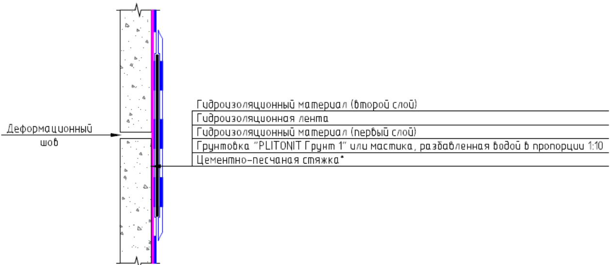
Рис.33.3. Конструктивный разрез №3.
