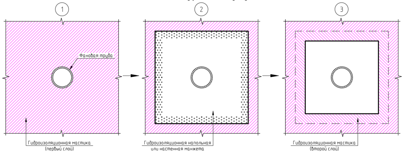
Рис.33.4. Последовательность нанесения гидроизоляционной манжеты.
