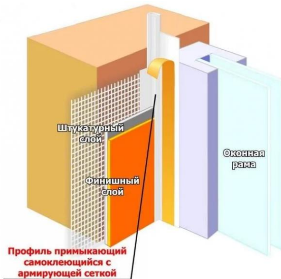
Рис.25. Профиль примыкающий с армирующей сеткой
