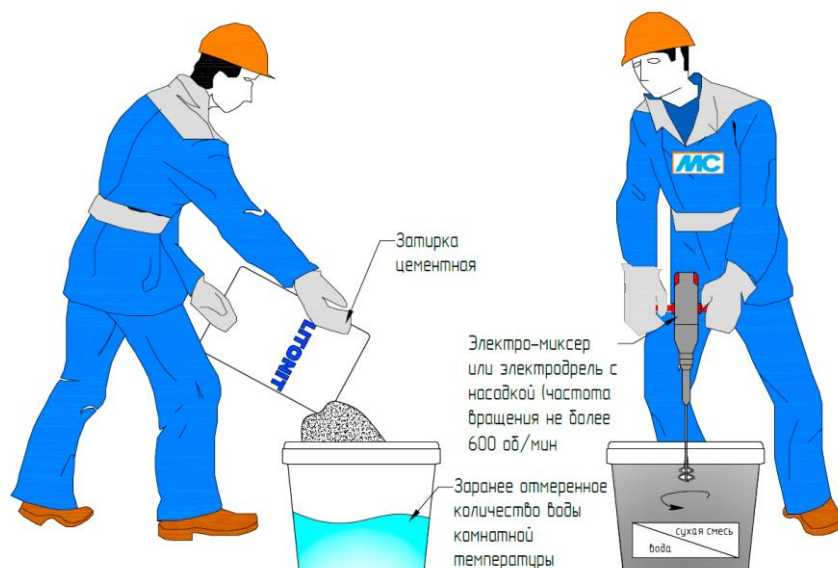
Рис. 38. Приготовление состава
