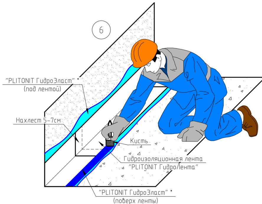
Рис.34.1. Последовательность работ (на стенах работа в аналогичном порядке), где: 1 - проверка ровности основания контрольной рейкой (аналогично для горизонтальной поверхности); 2 – размешивание емкости с мастикой; 3 – нанесение первого слоя мастики, разбавленной водой в пропорции 1:10, на основание; 4 – нанесение гидроизоляции на поверхность (аналогично для горизонтальной поверхности); 5 – укладка гидроизоляционной ленты на поверхность, предварительно обработанную «PLITONIT ГидроЭласт» или «PLITONIT WaterProof Standard»; 6 – поверхностная обработка ленты мастикой «PLITONIT ГидроЭласт» или «PLITONIT WaterProof Standard».
