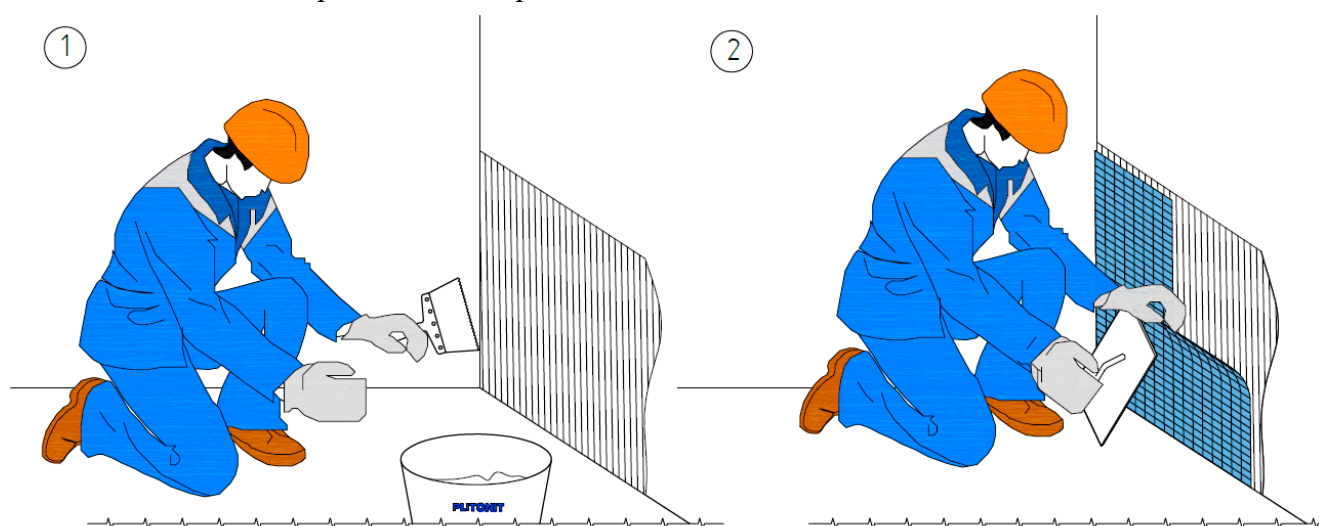
Рис. 36. Организация работ по приклеиванию мозаики
