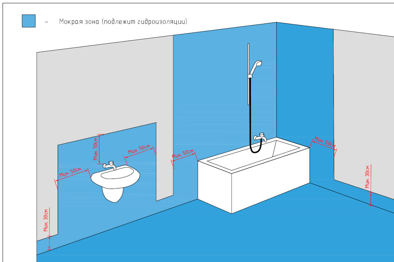
Рис. 34.2 Мокрые зоны внутри влажных помещений, подлежащие гидроизоляции.
