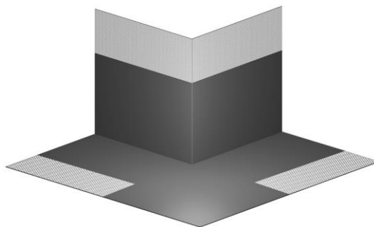
Рис.15. Гидроизоляционный угол «PLITONIT ГидроЛента угол внешний 270°».
