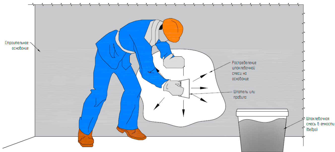
Рис. 32. Организация работ по нанесению шпаклевочной смеси
